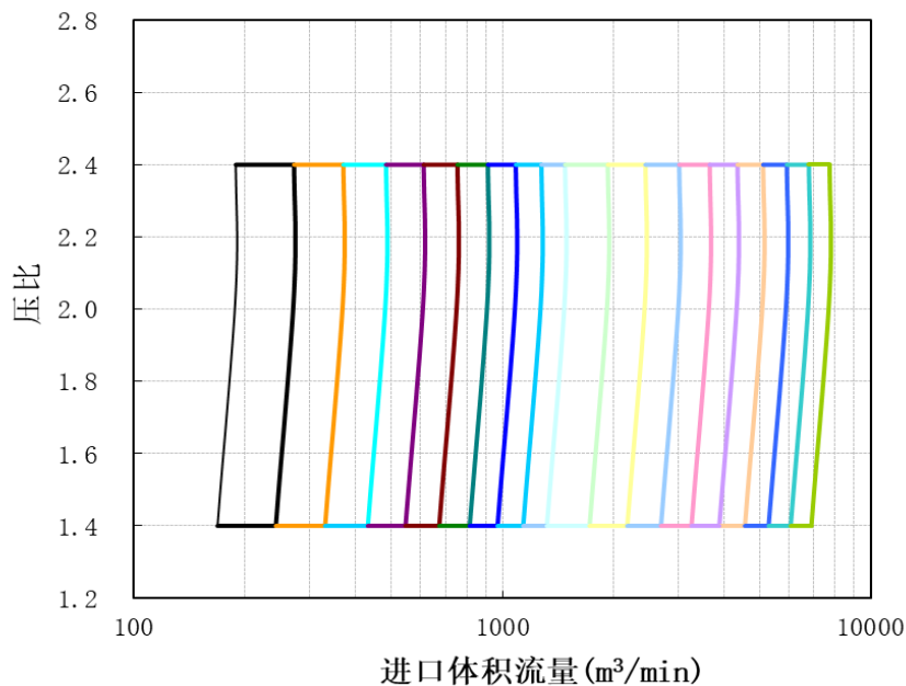
三一环保水蒸汽压缩机特性范围图谱
